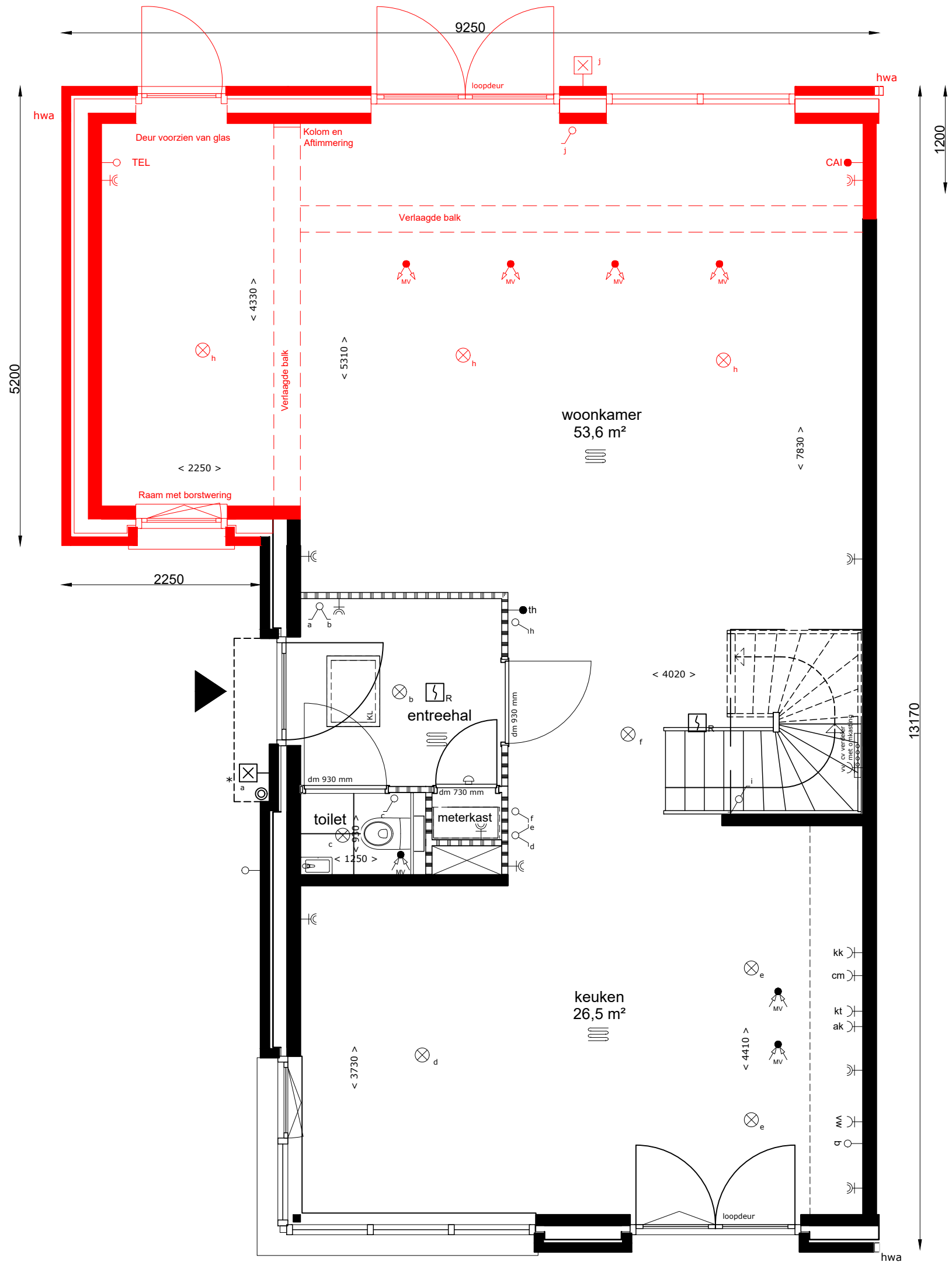
Begane grond
